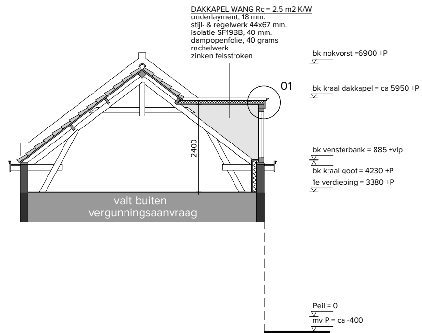
doorsnede nieuw
