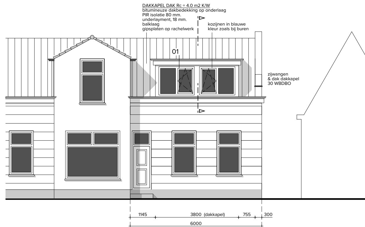
gevelaanzicht nieuw
